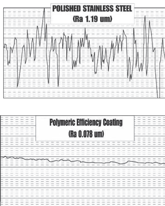
圖5：拋光不銹鋼(上)和新研發的高分子效率塗層(下)的粗糙度比較 ([5]Talysurf Surface Inspection, Leeds University, 1989)
